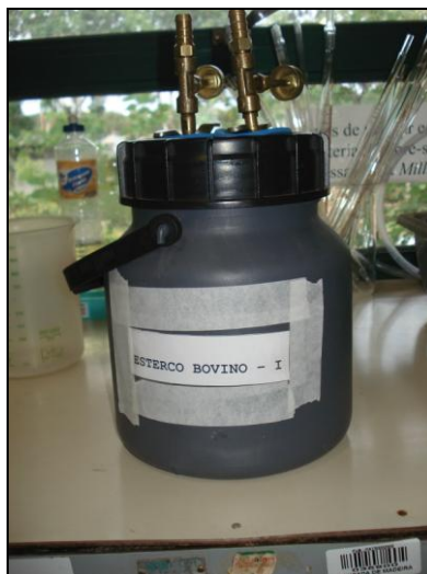
Figura 4.2: Recipiente utilizado como bioreator na pesquisa.
