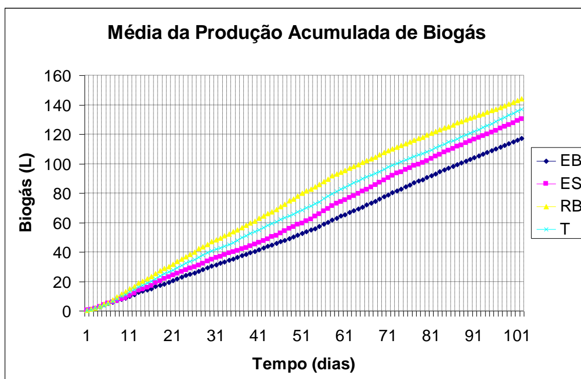
Figura 5.1: Média da produção acumulada de biogás nos bioreatores.
